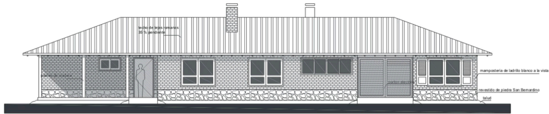
CASA A FACHADA PRINCIPAL
