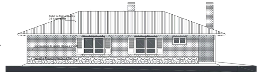
CASA A FACHADA LATERAL
