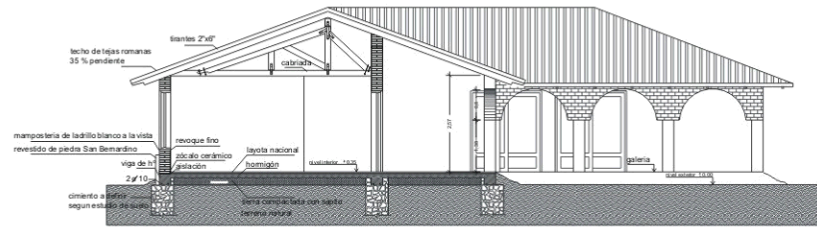
CASA A CORTE B-B
