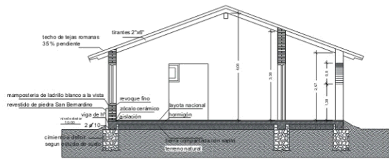
CASA A CORTE C-C
